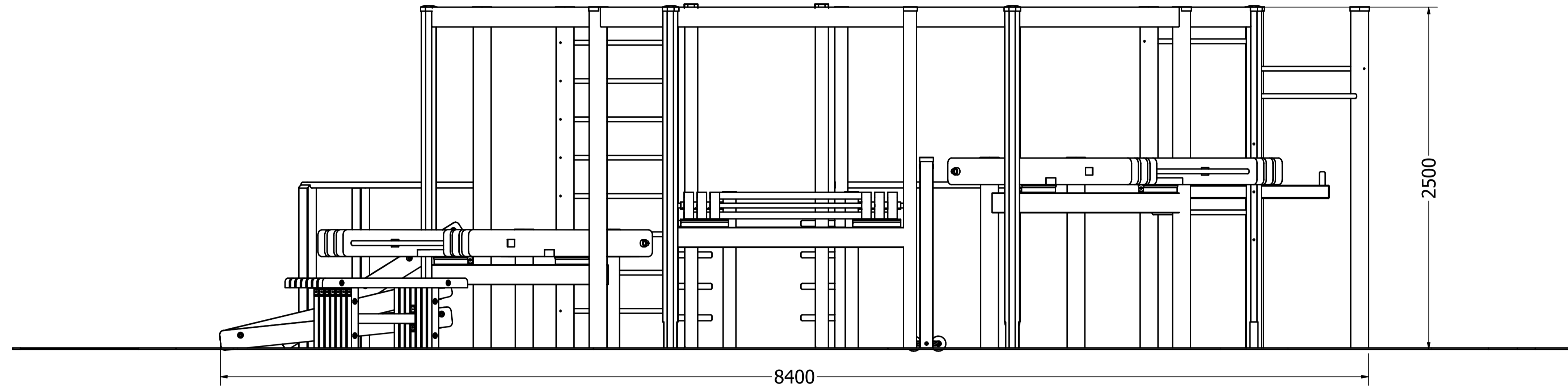
TO.1 Oktagym Vänster sida skala 1:20
