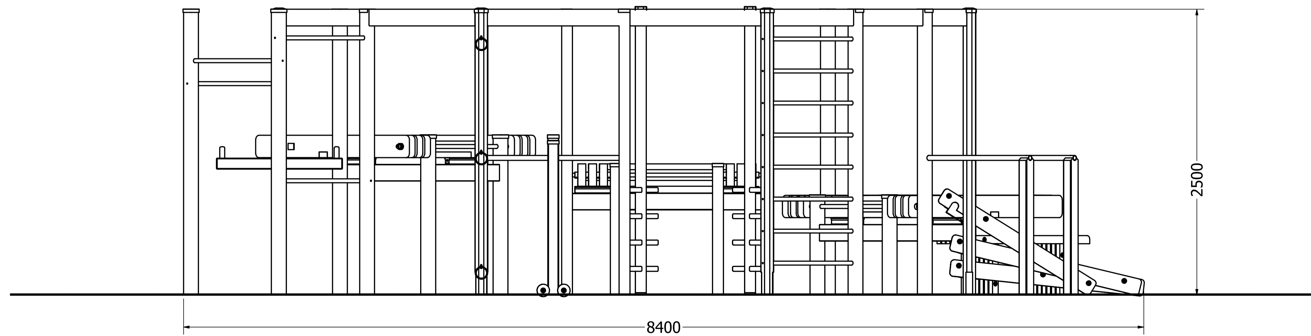
TO.1 Oktagym Höger sida skala 1:20
